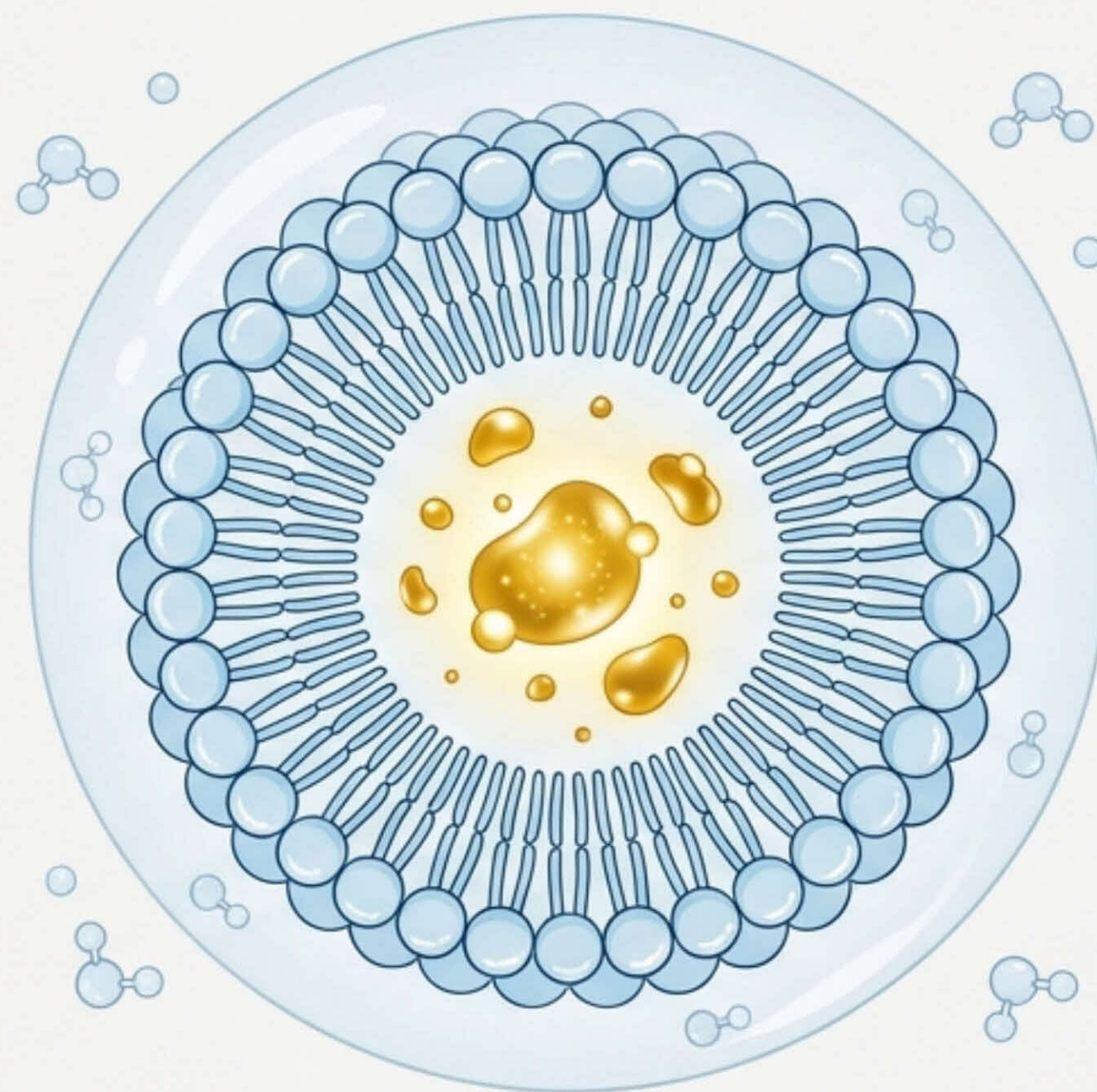
ミセル（球体）
